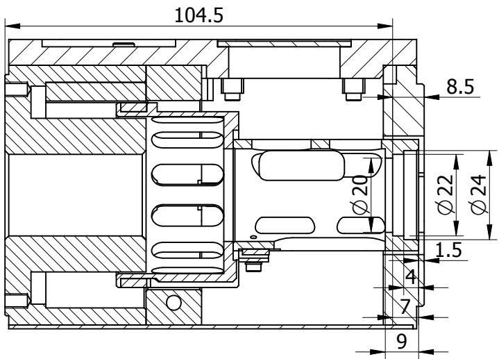
剖面 A-A
